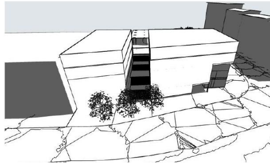
Faille
